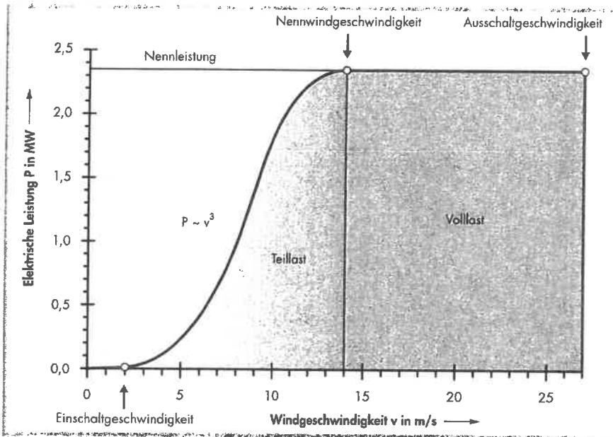
Bild 5. Typische Kennlinie einer modernen Windenergieanlage.
